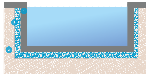
1 Structure béton armé 2 MISAPOR 3 Terrain naturel
