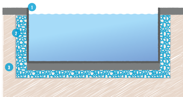
1 Structure inox 2 MISAPOR 3 Terrain naturel
